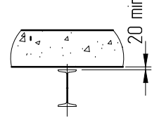
Е-Е (1:20)
