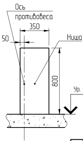
М (1:20)
