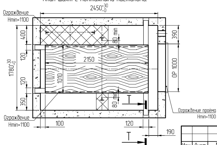
План шахт с монтажными настилами.
